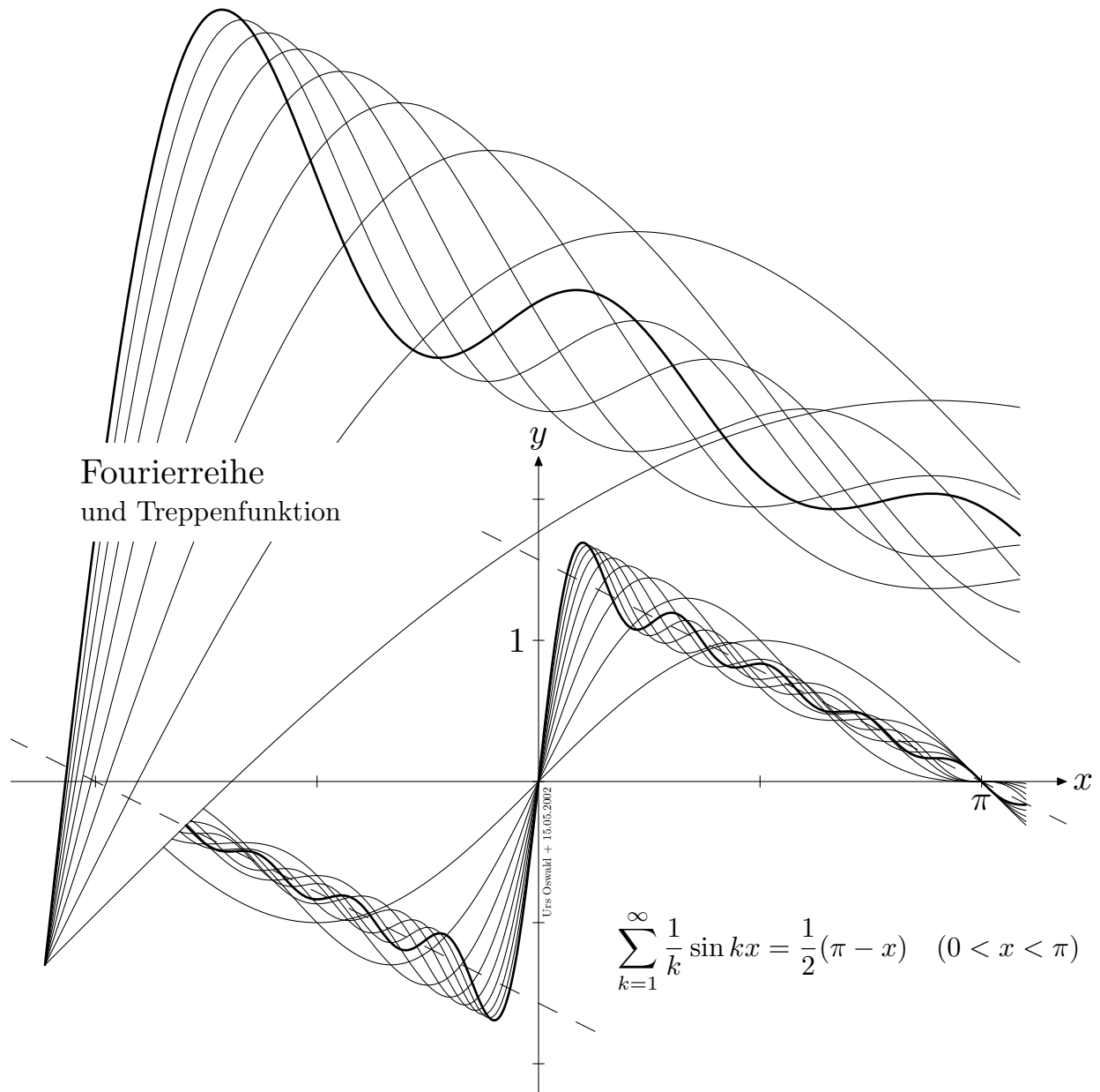
Fourier.eps
