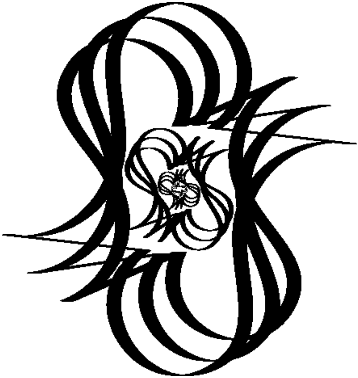
Lissajoux.png
